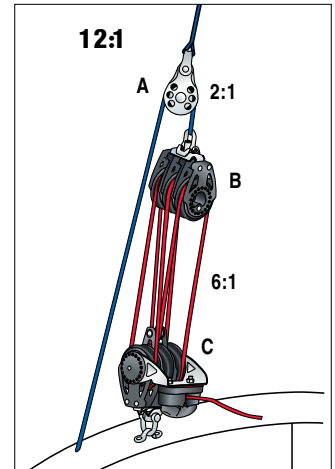
12:1 Kaskade: Variante zu 1: Über einen Draht-Block am Ende des Stags wird ein flexibler Draht geführt: diese 12:1 Übersetzung erhöht die gesamte auf 6:1 Übersetzung.
