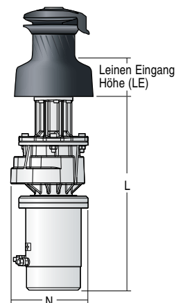
ELEKTRISCH-VERTIKAL
