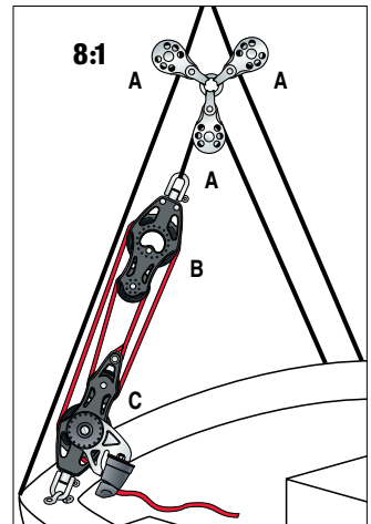
8:1 Geteiltes Achterstag, Kaskade: Eine stärker übersetzte Variante von 3. Ein Draht läuft über den Drahtblock, für eine gesamte Übersetzung von etwa 8:1.
