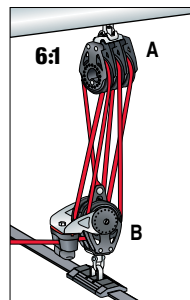
6:1 Direkt: Schiffe mit Grosssegelflächen bis 35m 2 (375 ft 2 ) setzen oft eine 6:1 Talle ein.
