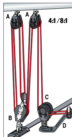
4:1/8:1 Dreh-Basis: Dieses System ist dem 3:1/6:1 Dreh-Basis ähnlich; 4:1/8:1 für mehr Zugkraft.
