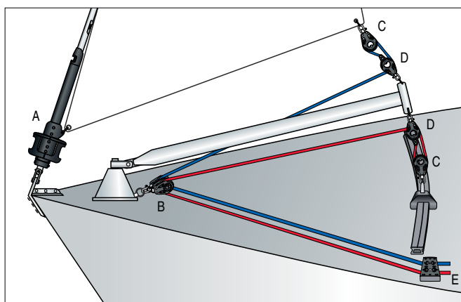
Selbstwender mit Fockbaum: Selbstwende-Fock und Stagsegel arbeiten bestens mit Roll-Reff System und Fockbaum. Zwei Schoten kontrollieren die Fock gegenüber dem Baum, bzw. den Baum.
