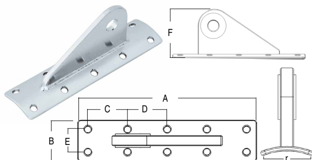
RUNDER BAUMBESCHLAG
