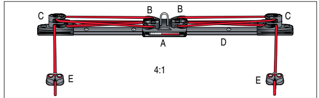
4:1 Klemme abseits: Wo der Traveller vor dem Schiebeluk angebracht wird, ist es zweckmässig, die Klemmen am achterlichen Ende des Kajütdachs zu plazieren.
