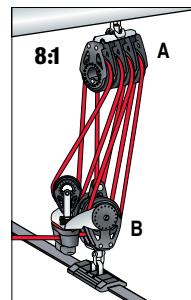
8:1 Strand-Kat: Diese 8:1 Talle ist geeignet für Grossschot Lasten auf Strand-Kats bis 6m (20').
