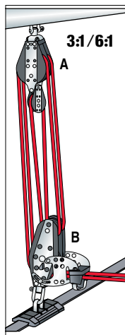
3:1/6:1: Mit diesem 3:1/6:1 System kann der Grossschoter praktisch von überall her die Schot bedienen. Ideal für Sport-Boote.
