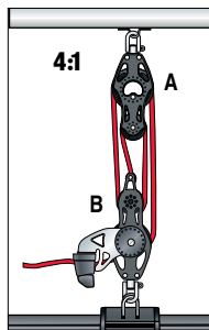
4:1 Violin: Das gebräuchlichste Grossschot-System auf Schiffen unter 8.5m (28') ist eine 4:1 Talle.
