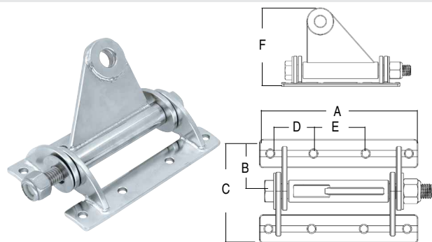
EINSTELLBARER BAUMBESCHLAG
