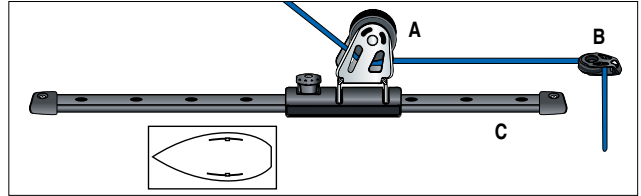
Pinstop Schlitten: Ein Pinstop Schlitten auf Kugellager-Schiene kann dort empfohlen werden, wo die Option eines Kugellager-Wagens für später offen bleiben soll.
