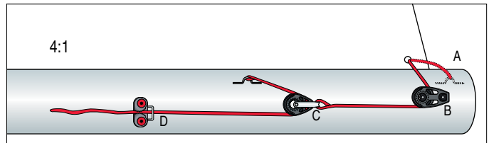
4:1 Kaskade extern: Dieses einfache, aussen liegende System verwendet zwei 2:1 Taljen, um eine 4:1 Übersetzung zu erzielen.
