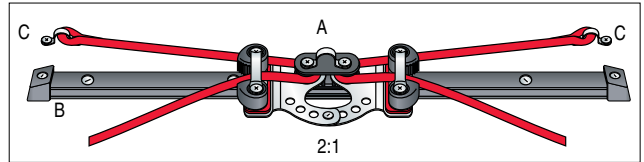
2:1 Klemme auf Wagen: Bei diesem System sind die Klemmen auf Armen, die im Winkel auf den Trimmer eingestellt werden.
