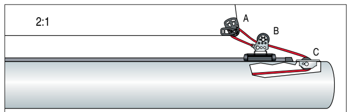
2:1 Rollbares Grossegel: Grossegel, die in den Mast gerollt werden, haben ein offenes Unterliek und normalerweise am Schothorn einen kugelgelagerten Schlitten, der über die ganze Länge des Grossbaums läuft. Die Ausholleine beginnt am Schlitten, läuft durch den Block am Schothorn, über die Scheibe auf dem Schlitten in den Baum, und auf eine Winch.
