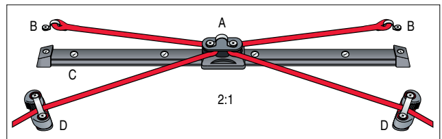
2:1 Klemme abseits: Beliebte auf Flush-Deck Booten ist dieses 2:1 System; auf der J/24 etwa sitzt die Crew aussenbords vom Traveller.
