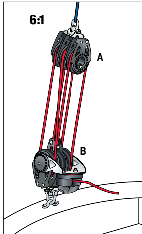
6:1 Direkt: Dieses einfache 6:1 System wird auf kleinen Fahrten-Schiffen mit einzelner Achterstag eingesetzt.
