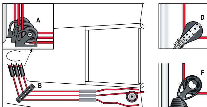
3 Fallen: Grössere Schiffe verwenden spezielle Mastfuss Umlenk-Blöcke. Die Falle führen durch Umlenker nach achtern zu Stoppern und Winschen. Aufgestellte Blöcke auf einer Basis werden manchmal vorgezogen wegen ihrer allseitigen Beweglichkeit; aber sie halten die Leine weniger nah am Deck als die spezialisierten Mastfuss-Blöcke.
