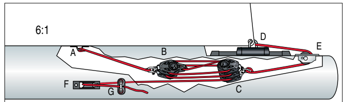
6:1 Intern: Ein 6:1 interner Strecker ist verbreitet auf kleineren bis mittleren Offshore Booten; sie schlagen das Schothorn des Grossegels an einem Traveller Schlitten an.
