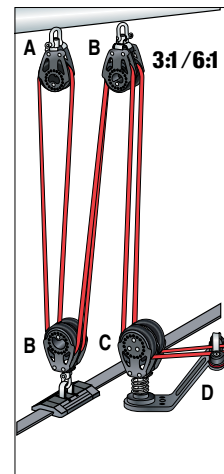
3:1/6:1 Dreh-Basis: Dieses 3:1/6:1 System ist grossartig für Sport-Boote.
