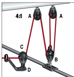
4:1 Dreh-Basis: Führt man die Grossschot vom Traveller weg auf einen Ratschblock auf einer Basis, kann man die Grossschot einstellen, ohne den Schlitten nach Luv zu ziehen. Dies tendiert dazu, das Liek leicht zu schliessen; dem kann mit konkav gebogener Schiene entgegen gewirkt werden.
