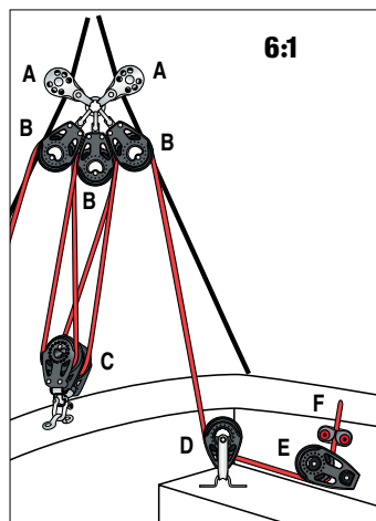
6:1 Geteiltes Achterstag, zwei Enden: Dieses System für geteiltes Achterstag hat zwei Enden, die unmittelbar vor dem Steuermann von beiden Seiten bedient werden können.
