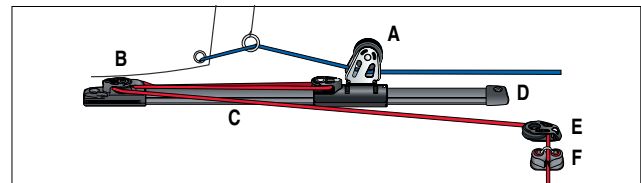
Barberholer: Dieses System niedriger Bauweise ist für Renn-Yachten mit nicht überlappendem Fock, wie etwa die Farr® 40 und One Design 35. Ein 'Einholer' kontrolliert den Spalt.
