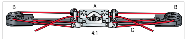
Automatik: Der patentierte Mechanismus lässt den Wagen nach luv holen, ohne die Leeklemme vorher zu lösen. Nach der Wende bleibt der Schlitten stehen, und kann dann ins neue Luv geholt werden.
