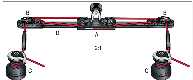
2:1 mit dedizierter Winch: Nehmen Sie dieses System für grosse Schiffe, wo der Traveller über die Winch eingestellt wird.
