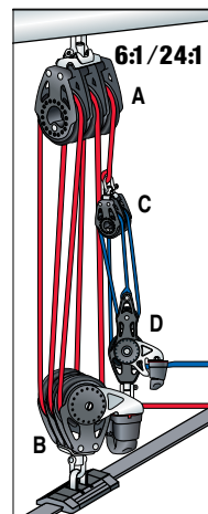
6:1 / 24:1 Kaskade: Dieses 6:1/24:1 System wurde entwickelt für Yachten mit Grosssegel-flächen bis zu 25.5m 2 (275 ft 2 ) und Aufhängung an der Nock.
