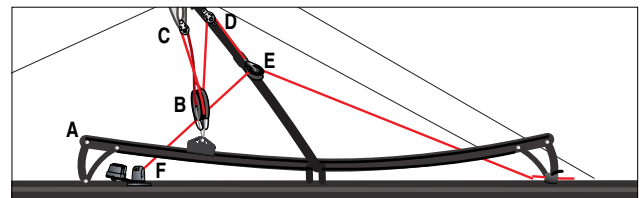
Crossbow Schwenkenden Fock Traveller: Der Crossbow ist ein Selbstwende Fock System für Hochleistungs-Jollen, Skiff und Katamaran unter 6m (20').
