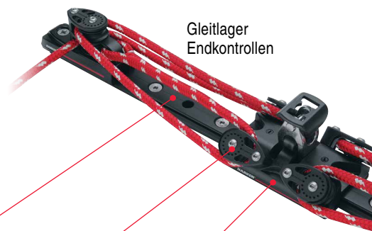
Kugelgelagerte Endkontrollen
